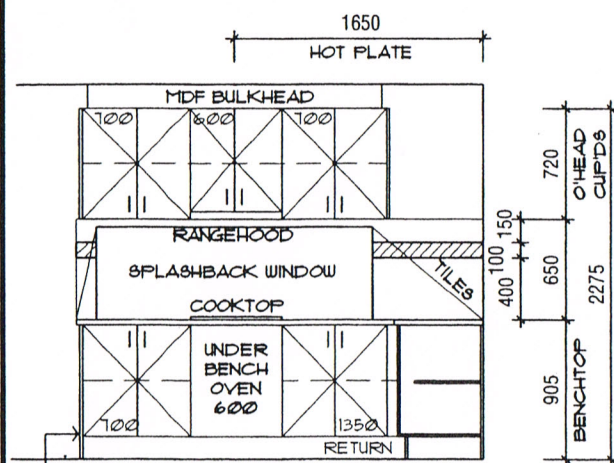
ELEVATION 1
