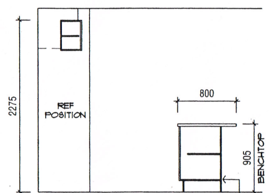
ELEVATION 3
