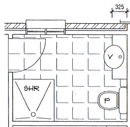
ENSUITE FLOOR PLAN
