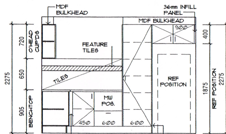
ELEVATION 2
