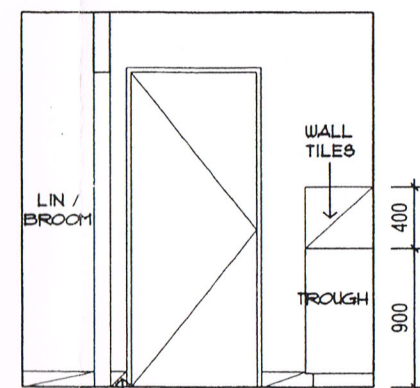
ELEVATION 1
