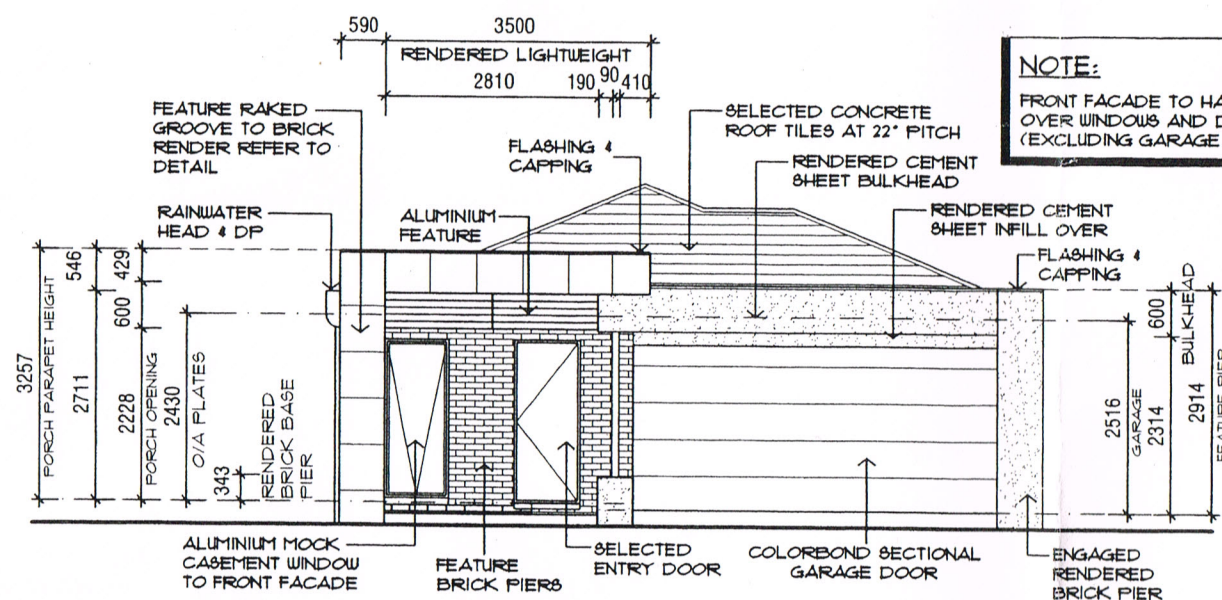
ELEVATION A
