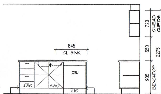
ELEVATION 4
