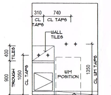
ELEVATION 2
